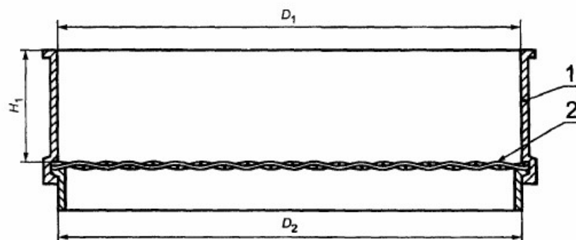
1 — обечайка (рамка); 2 — сетка из металлической проволоки
